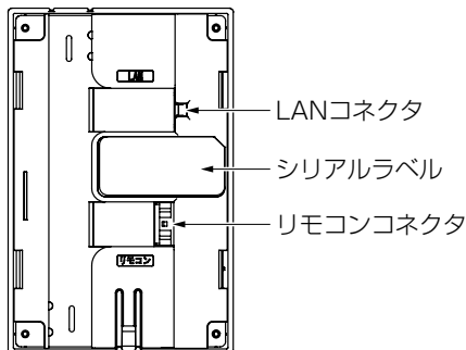
<裏面>
