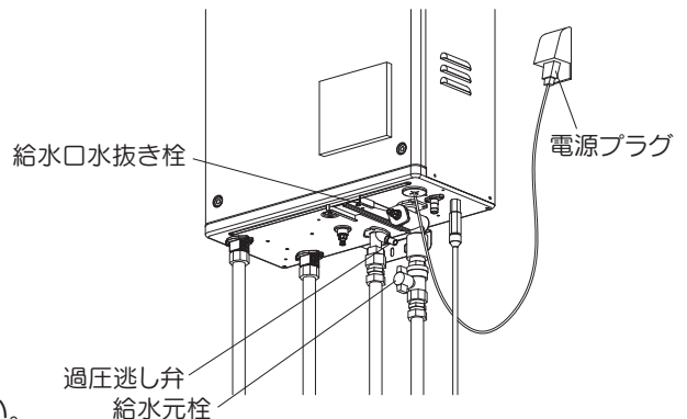
壁掛けタイプ (CKX-G472KSAF・CKX-G472KSAFF)
