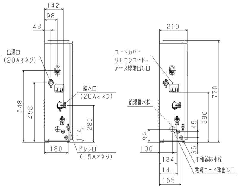
配管位置
