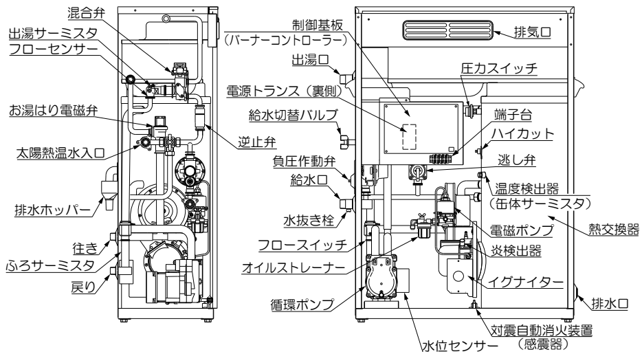
●構 造 図
